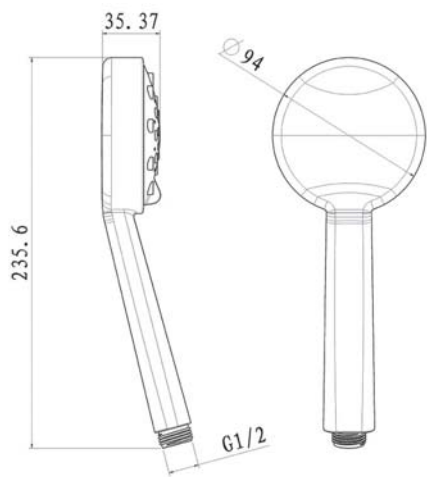
арт. 5035 Swedbe Calypso Лейка душевая
