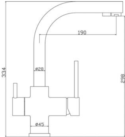
апт. 8147 Swedbe Selene Plus Смеситель для кухни с каналом для фильтрованной воды
