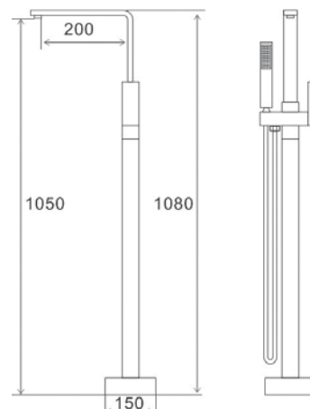
арт. 4005 Swedbe Spira Смеситель напольный
