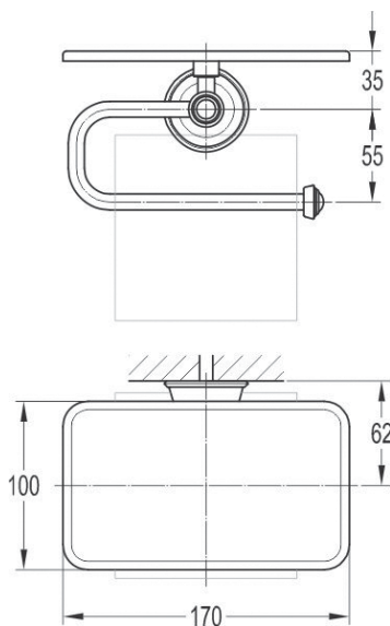
арт. 2544 Swedbe Terracotta Art Держатель для туалетной бумаги
