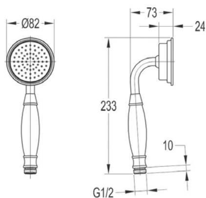
арт. 2529 Swedbe Terracotta Art Лейка душевая
