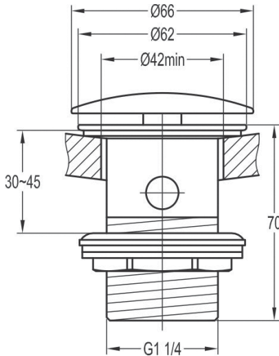
арт. 2563 Swedbe Terracotta Донный клапан
