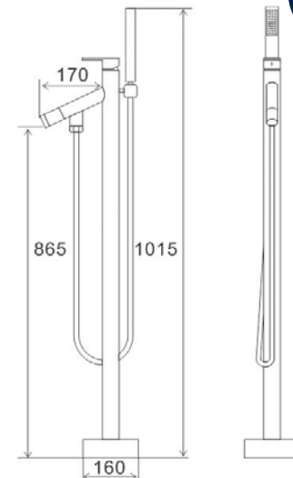
арт. 4010 Swedbe Spira Смеситель напольный
