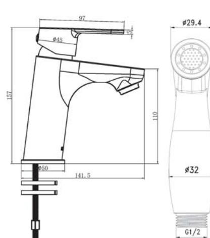
арт. 1830 Swedbe Olymp Смеситель для ванны
