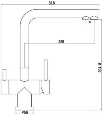
апт. 8144 Swedbe Selene Plus Смеситель для кухни с каналом для фильтрованной воды
