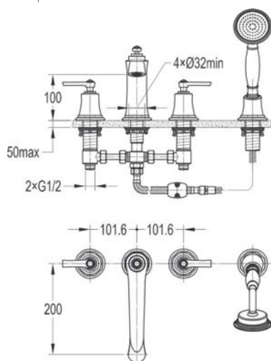
арт. 2507 Swedbe Terracotta Art Смеситель для ванны с душевой лейкой на 4 отверстия
