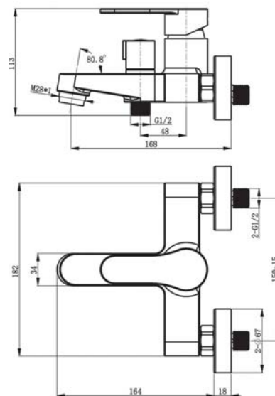
арт. 2130 Swedbe Atlas Смеситель для ванны
