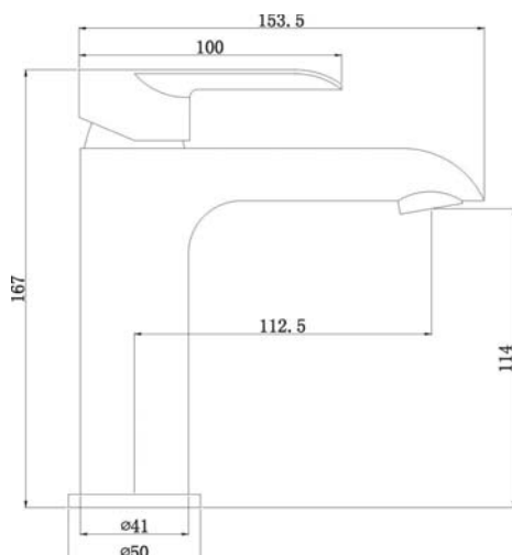
арт. 8010 Swedbe Hermes Смеситель для раковины
