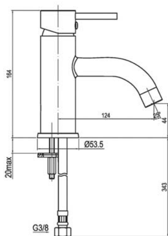
арт. 1510 Swedbe Jupiter Смеситель для раковины
