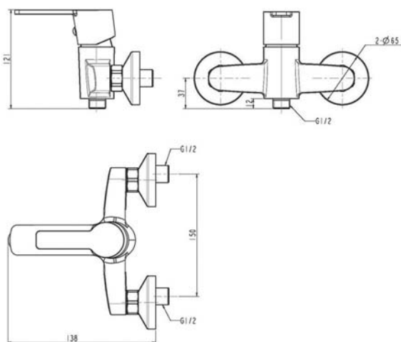
апр. 2020 Swedbe Kronos Смеситель для душа
