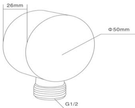
ар. 5506 Swedbe Platta Подсоединение шланговое
