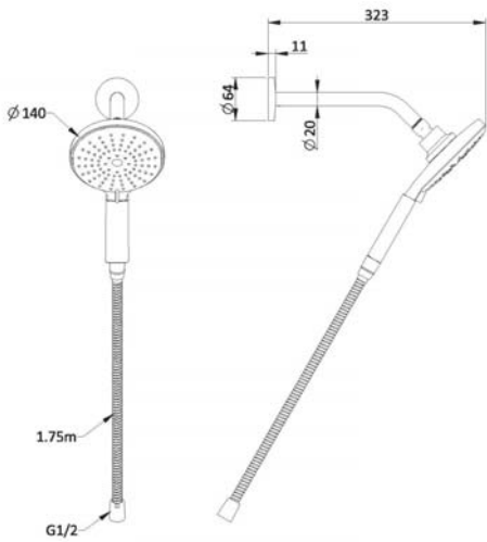
арт. 5013 Swedbe Calypso Комплект душевой с магнитным держателем
