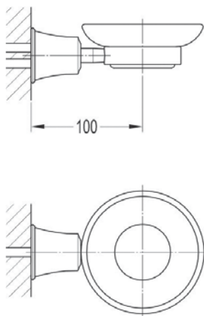
арт. 2542 Swedbe Terracotta Art Мыльница с держателем
