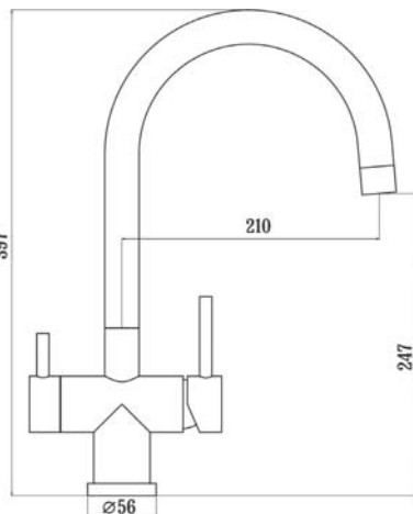
арт. 8042 Swedbe Selene Plus Смеситель для кухни с каналом для фильтрованной воды
