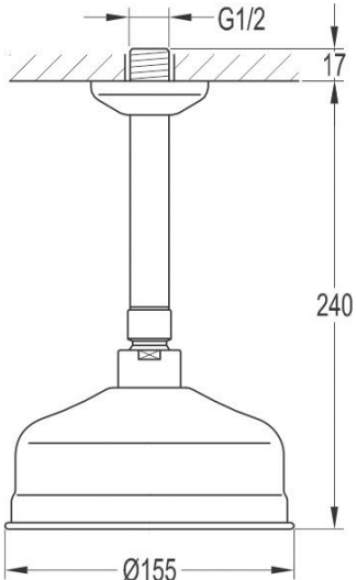
арт. 2555 Swedbe Terracotta Кронштейн душевой с верхним душем
