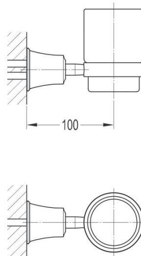
арт. 2541 Swedbe Terracotta Art Стакан с держателем
