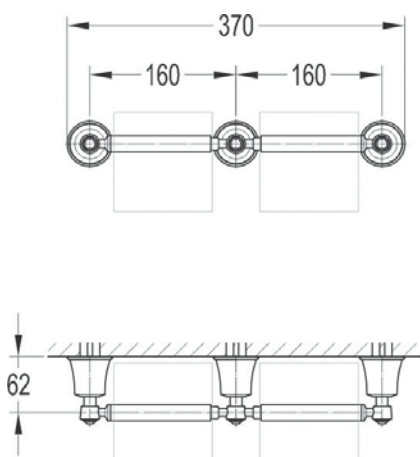
арт. 2545 Swedbe Terracotta Art Держатель для туалетной бумаги двойной
