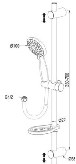
арт. 5010 Swedbe Harmony Комплект душевой
