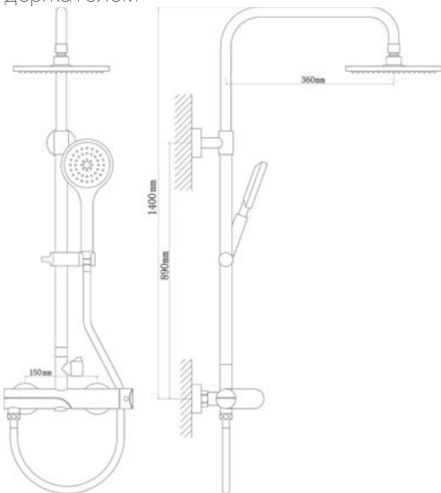
арт. 5002 Swedbe Hermes Семейный душ со смесителем
