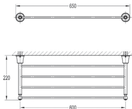
арт. 2539 Swedbe Terracotta Art Полотенцедержатель
