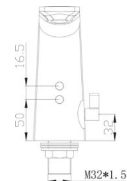
арт. 6020 Swedbe Europe Смеситель сенсорный для раковины
