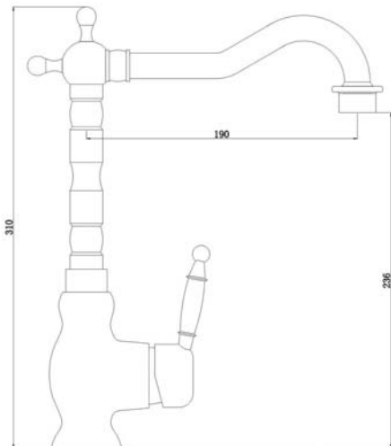
арт. 7141 Swedbe Selene Смеситель для кухни
