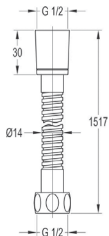
арт. 2535 Swedbe Terracotta Art Шланг душевой
