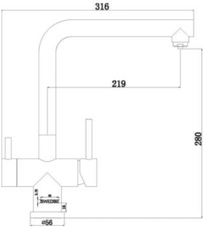
апт. 8145 Swedbe Selene Plus Смеситель для кухни с каналом для фильтрованной воды
