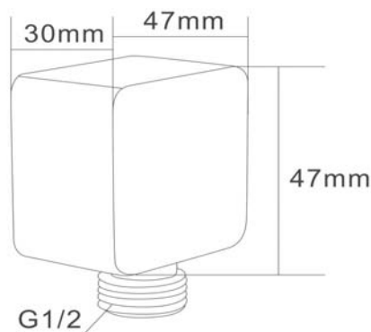
ар. 5508 Swedbe Platta Подсоединение шланговое
