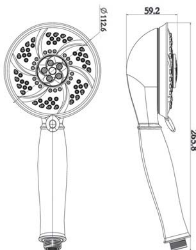
арт. 5014 Swedbe Calypso Лейка душевая
