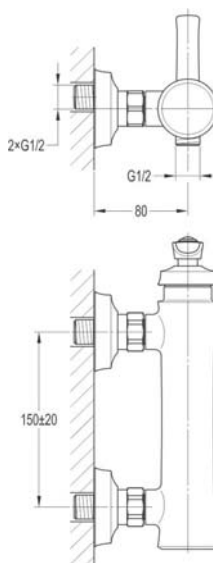
арт. 2509 Swedbe Terracotta Art Смеситель для душа
