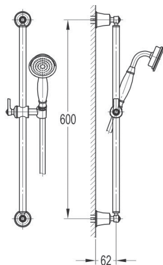
арт. 2533 Swedbe Terracotta Art Комплект душевой
