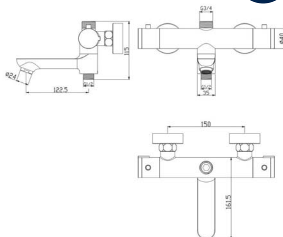
арт. 9042 Swedbe Hermes Смеситель термостатический для ванны с поворотным изливом
