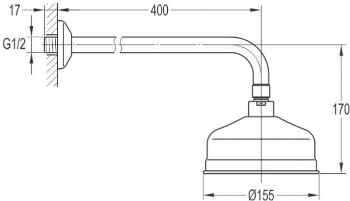
арт. 2558 Swedbe Terracotta Кронштейн душевой с верхним душем
