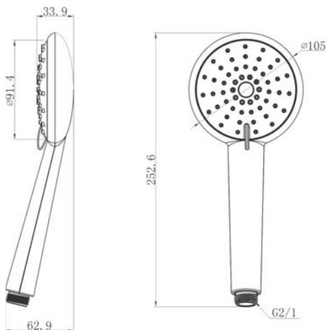
арт. 5050 Swedbe Calypso Лейка душевая
