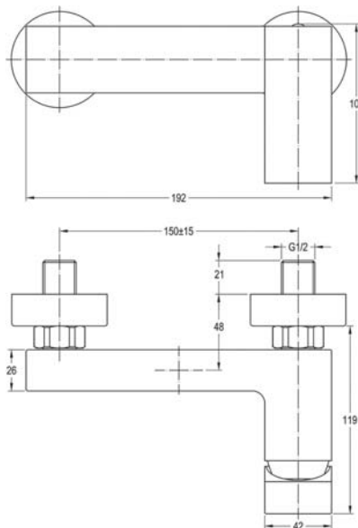
арт. 2420 Swedbe Velo Смеситель для душа
