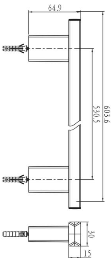
арт. 5044 Swedbe Calypso Стойка душевая
