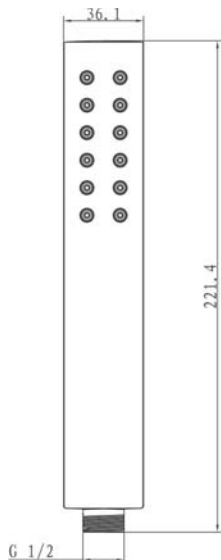
арт. 5039 Swedbe Calypso Лейка душевая
