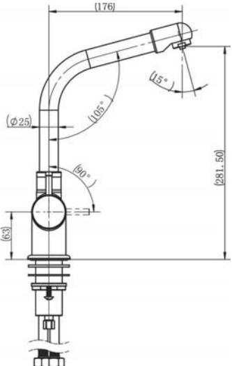
апт. 8140 Swedbe Selene Plus Смеситель для кухни с каналом для фильтрованной воды
