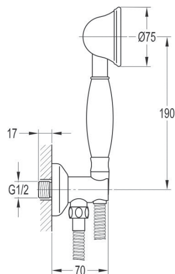
арт. 2556 Swedbe Terracotta Набор душевой
