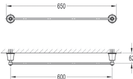
арт. 2537 Swedbe Terracotta Art Полотенцедержатель одинарный
