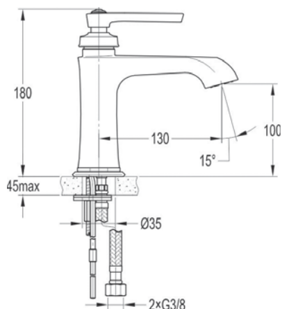
арт. 2500 Swedbe Terracotta Art Смеситель для раковины
