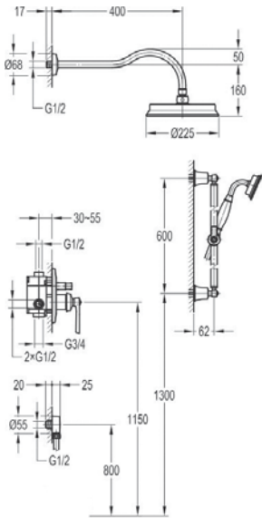
арт. 2515 Swedbe Terracotta Art Семейный душ со смесителем встраиваемый
