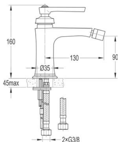
арт. 2505 Swedbe Terracotta Art Смеситель для биде
