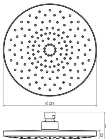
арт. 5047 Swedbe Calypso Верхний душ
