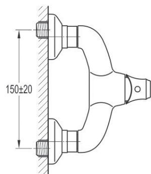
арт. 2552 Swedbe Terracotta Смеситель для душа
