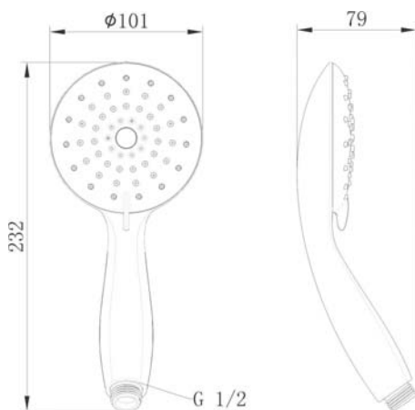
арт. 5049 Swedbe Calypso Лейка душевая
