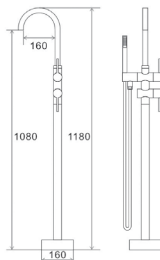
арт. 4004 Swedbe Spira Смеситель напольный
