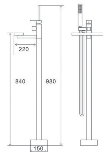
арт. 4008 Swedbe Spira Смеситель напольный
