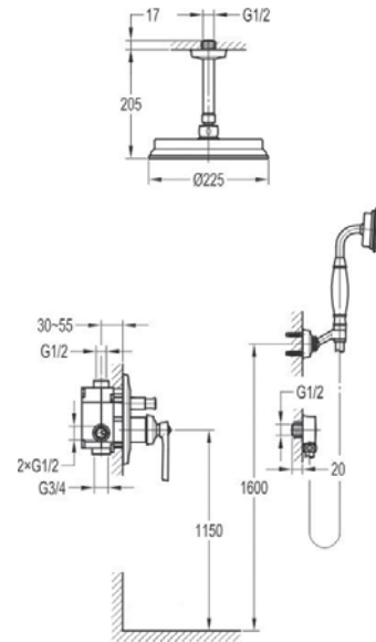
арт. 2516 Swedbe Terracotta Art Семейный душ со смесителем встраиваемый
