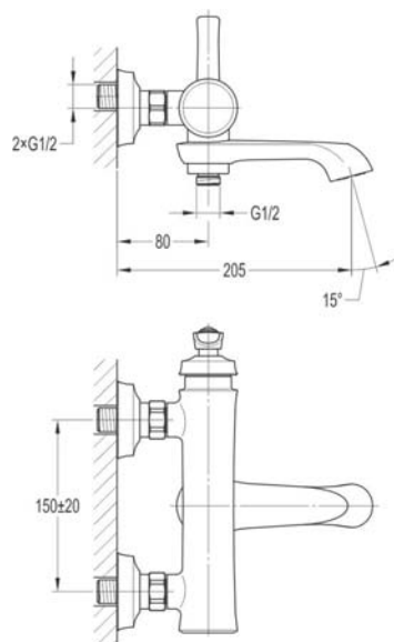
арт. 2510 Swedbe Terracotta Art Смеситель для ванны
