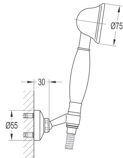
арт. 2562 Swedbe Terracotta Набор душевой
