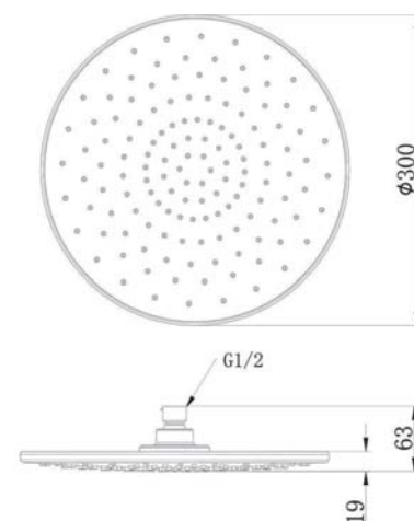
арт. 5046 Swedbe Calypso Верхний душ
