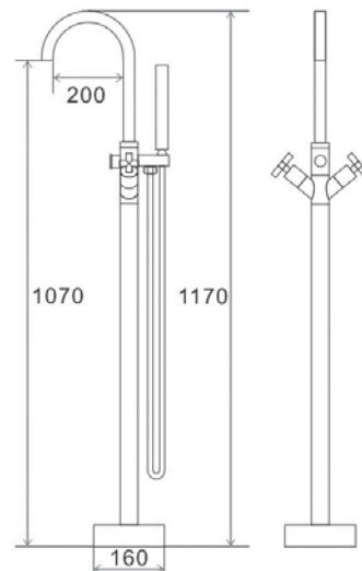
арт. 4002 Swedbe Spira Смеситель напольный
