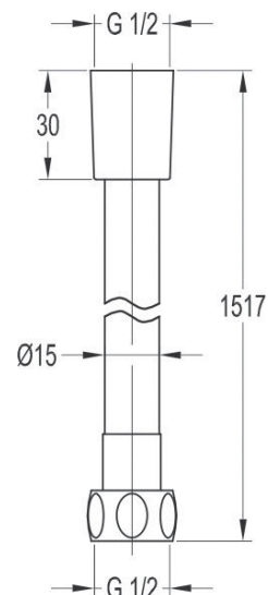
арт. 2530 Swedbe Terracotta Art Шланг душевой
