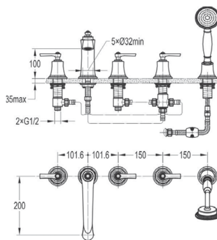
арт. 2508 Swedbe Terracotta Art Смеситель для ванны с душевой лейкой на 5 отверстий
