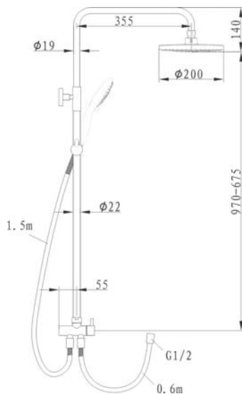
арт. 5006 Swedbe Harmony Семейный душ
