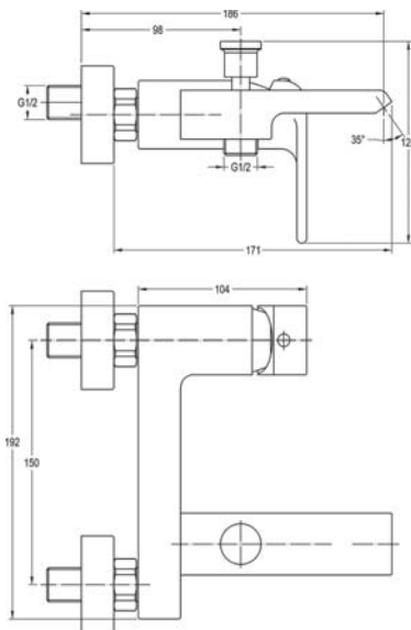
арт. 2430 Swedbe Velo Смеситель для ванны
