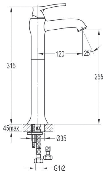
арт. 2549 Swedbe Terracotta Смеситель для раковины
