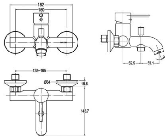
арт. 1530 Swedbe Jupiter Смеситель для ванны
