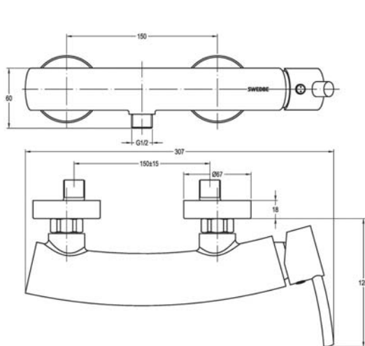
арт. 1420 Swedbe Saturn Смеситель для душа
