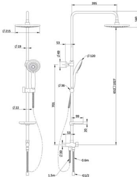
арт. 5007 Swedbe Calypso Семейный душ
