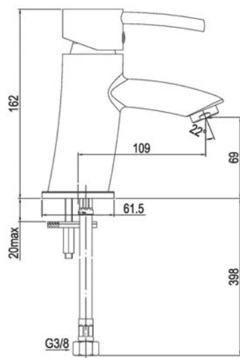
арт. 1410 Swedbe Saturn Смеситель для раковины
