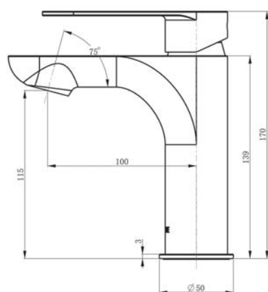
арт. 1110 Swedbe Vulcan Смеситель для раковины
