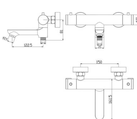
арт. 9045 Swedbe Mercury Смеситель термостатический для ванны с поворотным изливом
