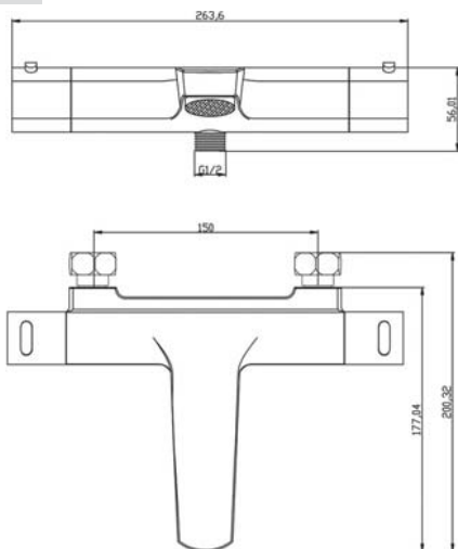
арт. 9063 Swedbe Mercury Смеситель термостатический для ванны
