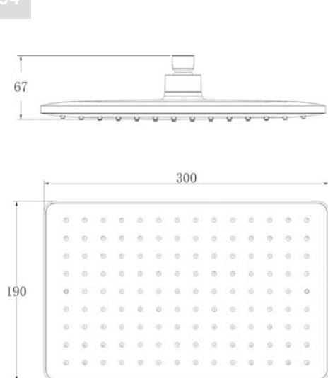
арт. 5041 Swedbe Calypso Верхний душ
