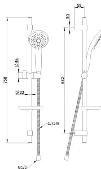
арт. 5011 Swedbe Calypso Комплект душевой
