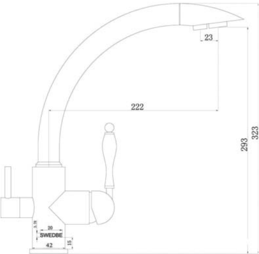
апт. 8044 Swedbe Selene Plus Смеситель для кухни с каналом для фильтрованной воды
