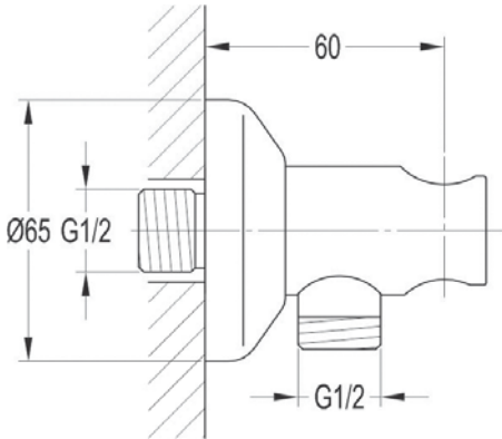
арт. 2559 Swedbe Terracotta Подключение шланговое с держателем
