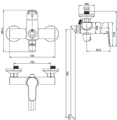
арт. 1850 Swedbe Olymp Смеситель для ванны с длинным изливом Z-формы
