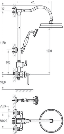
арт. 2511 Swedbe Terracotta Art Семейный душ со смесителем
