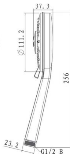
арт. 5042 Swedbe Calypso Лейка душевая
