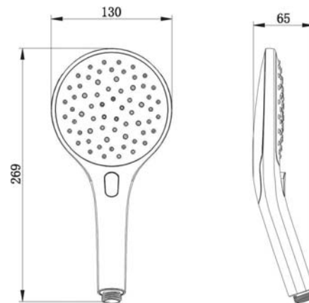
арт. 5015 Swedbe Calypso Лейка душевая
