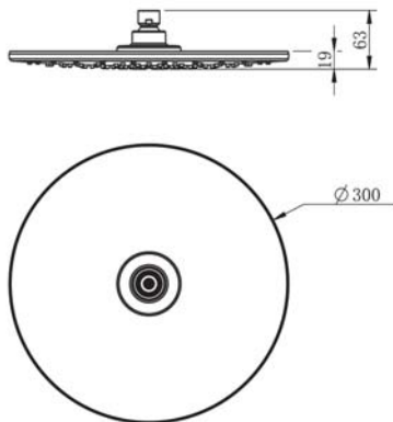
арт. 5036 Swedbe Calypso Верхний душ
