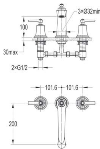
арт. 2506 Swedbe Terracotta Art Смеситель для ванны на 3 отверстия
