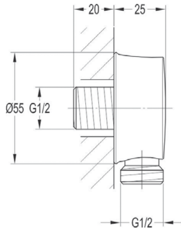
арт. 2526 Swedbe Terracotta Art Подключение шланговое
