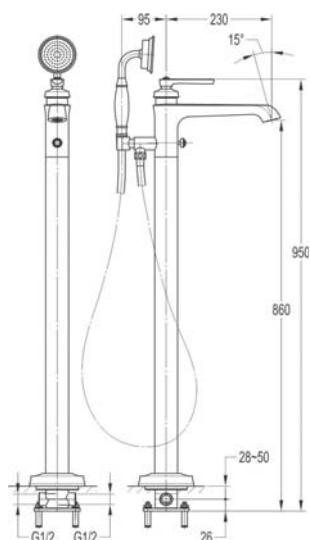
арт. 2514 Swedbe Terracotta Art Смеситель напольный с душевой лейкой
