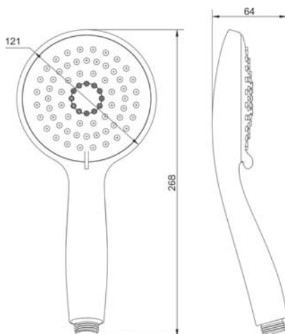
арт. 5016 Swedbe Calypso Лейка душевая
